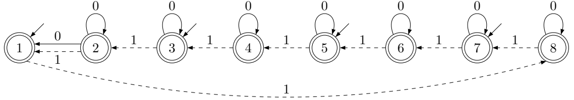
Obr. 3.2: FNA A_8
