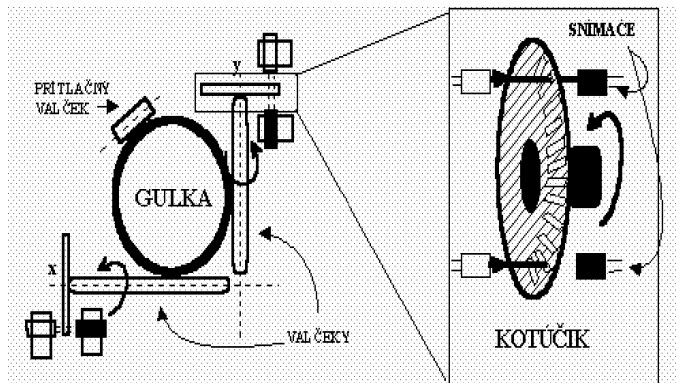
Obrázok 5.2: Princípy myši
