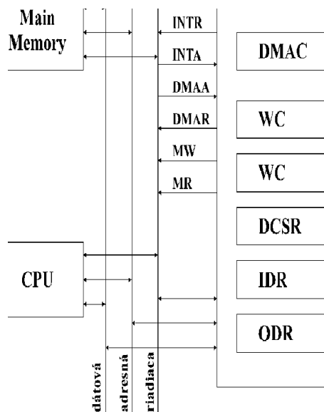
Obrázok 4.1: Schéma DMA-radiča
