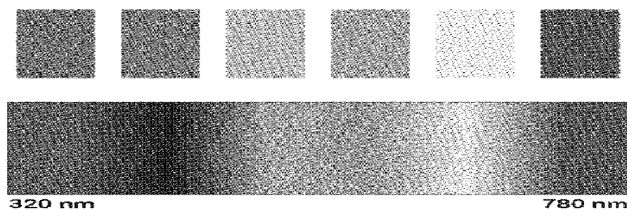
Obrázok 2.6: Farby spektra
