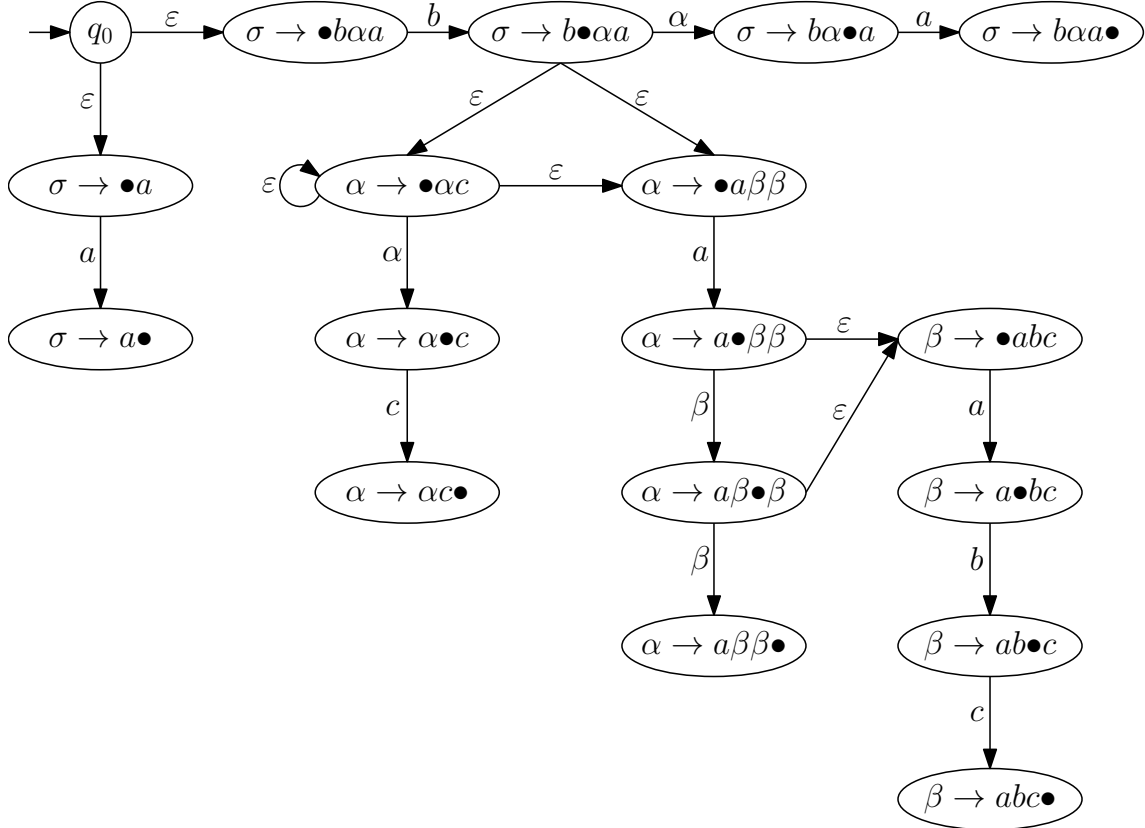
Obr. 1: Nedeterministický položkový automat \mathcal{N}_G zodpovedajúci gramatike G .
