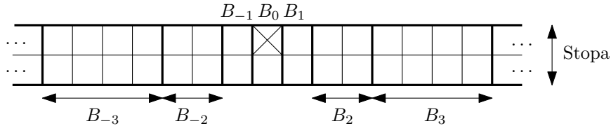
Obr. 2: Horizontálne členenie jednej zo stôp prvej pásky stroja A' .
