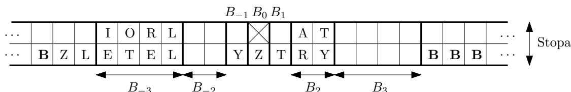
Obř. 3: Dvojřrovňovř stopa prvej přsky stroja A' reprezentujřcř slovo ZLETELIORLYZTATRY, přcřm hlava zodpovedajřcej přsky stroja A řřta druhř vřskyt přsmena Z.
