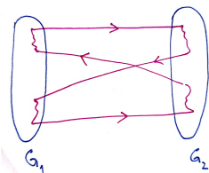
(a) Implikácia (a) \Rightarrow (c)
