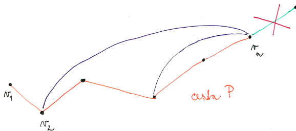
Obr. 4: Všetci susedia vrchola v_n ležia na ceste P
