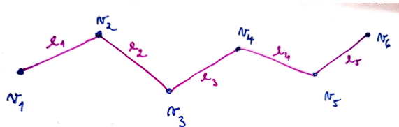
Obr. 2: Cesta dĺžky 5
