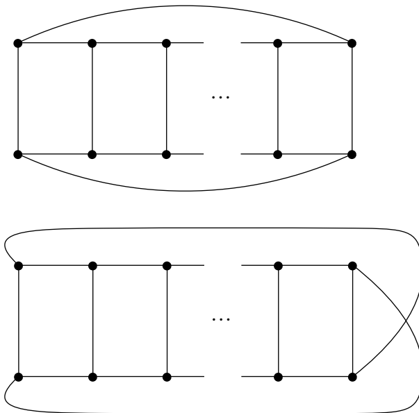
Obr. 6: Rebrík R_n a Skrútený rebrík S_n
