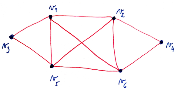
Obr. 3: Na obrázku je graf G . Postupnosť v_1v_2v_4v_6v_5 je cesta, v_1v_2v_6v_4v_2v_5 je ťah a v_1v_2v_4v_6v_2v_1v_3 je sled v grafe G .
