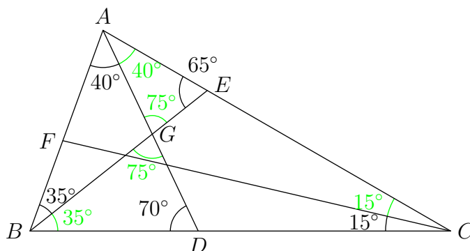
Obr. 2.18: Náčrt k úlohe 2.6.4, dopyčítané uhly sú zelené.
