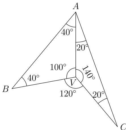
Obr. 2.2: Náčrt k úlohe 2.1.1
