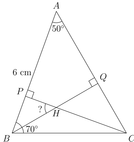
Obr. 2.1: Náčrt k úlohe 2.1.1
