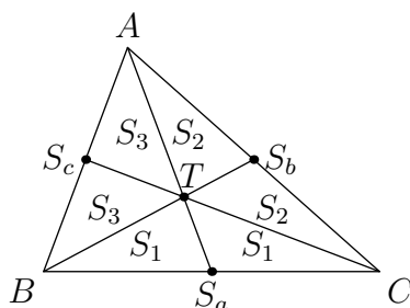
Obr. 2.16: Šesť trojuholníkov s rovnakým obsahom
