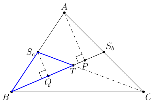
Obr. 2.17: Náčrt k inému dôkazu (ii)
