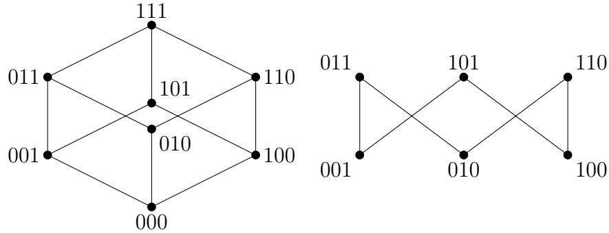
Obr. 2.1: Hasseho diagramy
